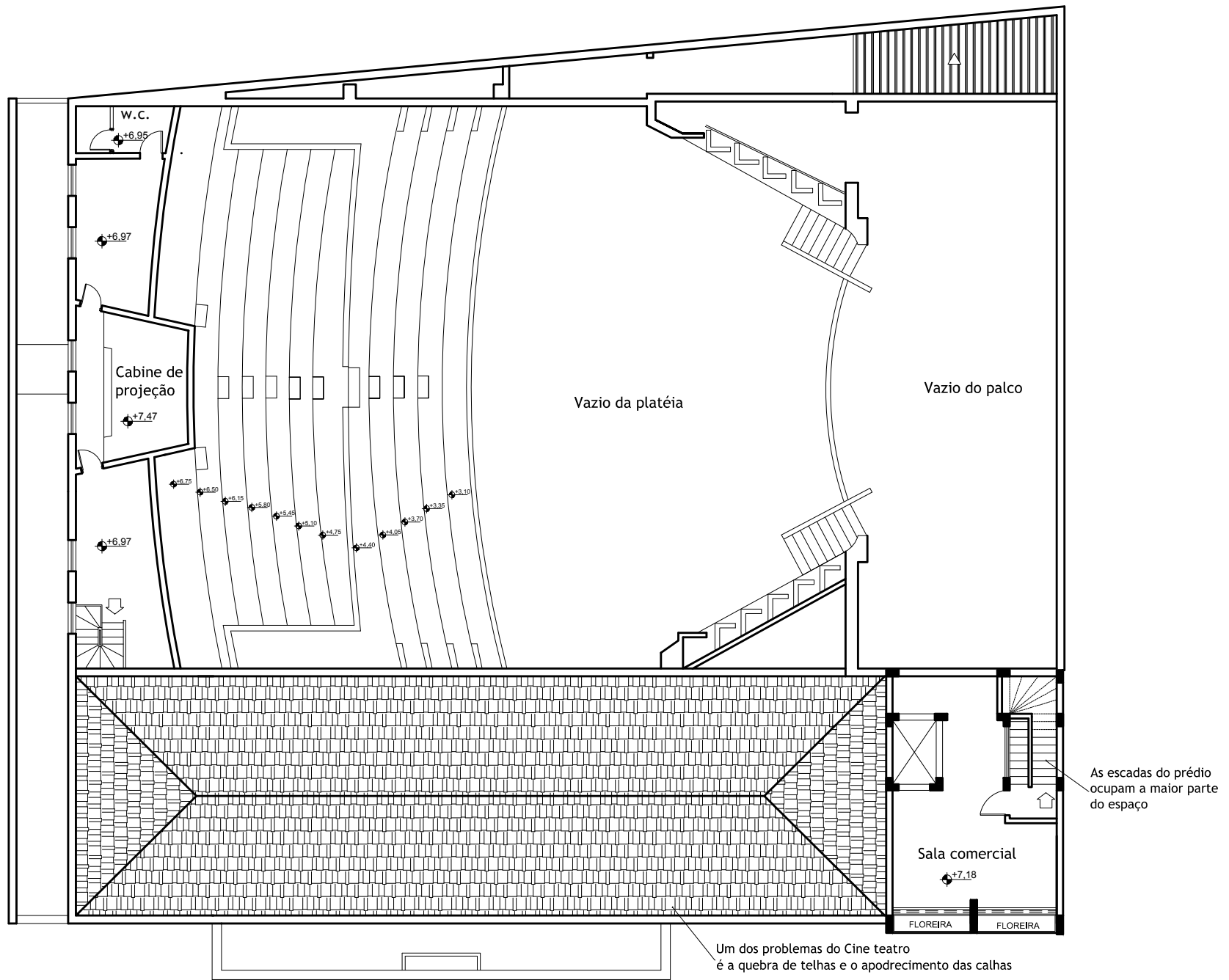
Planta Baixa Cine Teatro e Lemat-2. Pav. esc:1/200
